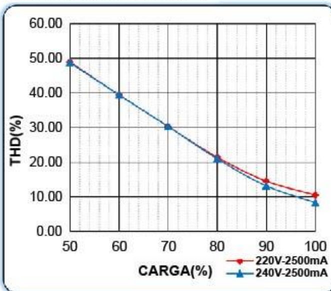
Distorsión armónica Vs Carga
