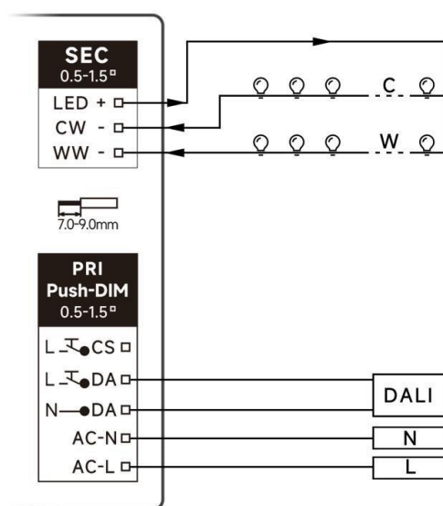
Conexión con DALI
