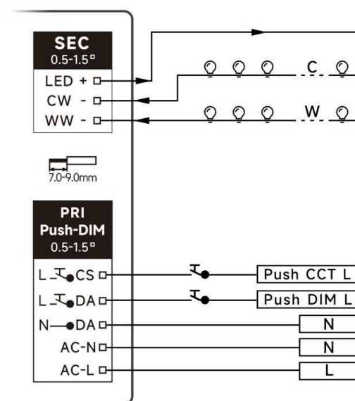
Conexión con pulsador
