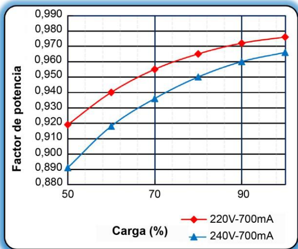
Características de factor de potencia
